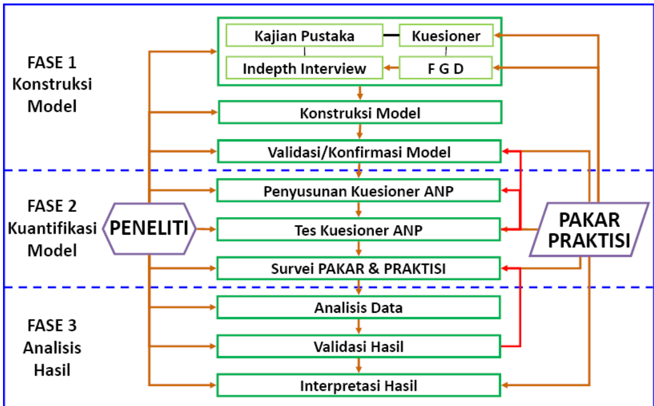
Gambar 3.1 Tahapan Penelitian
