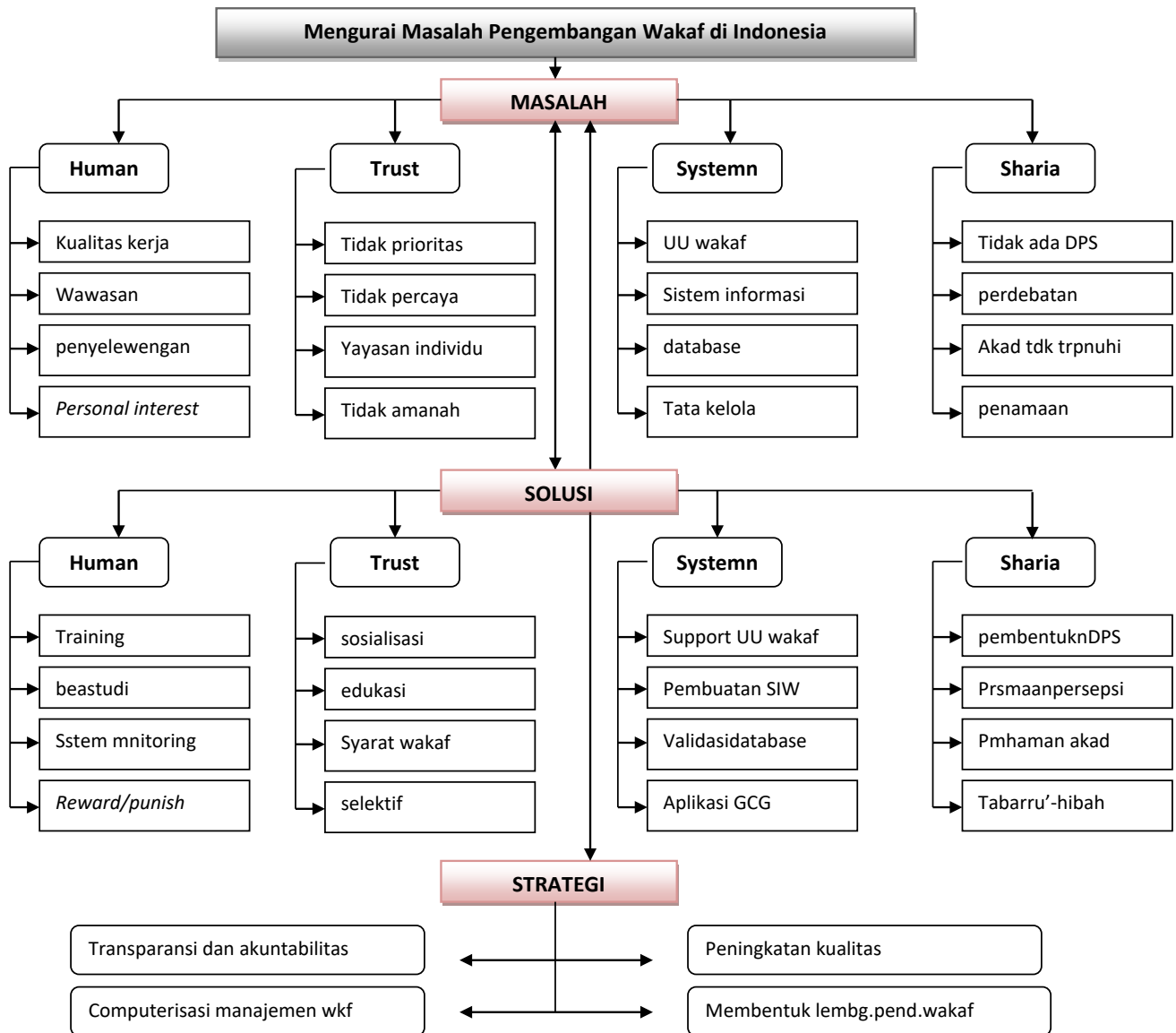
Gambar 4.1. Model Jaringan ANP
